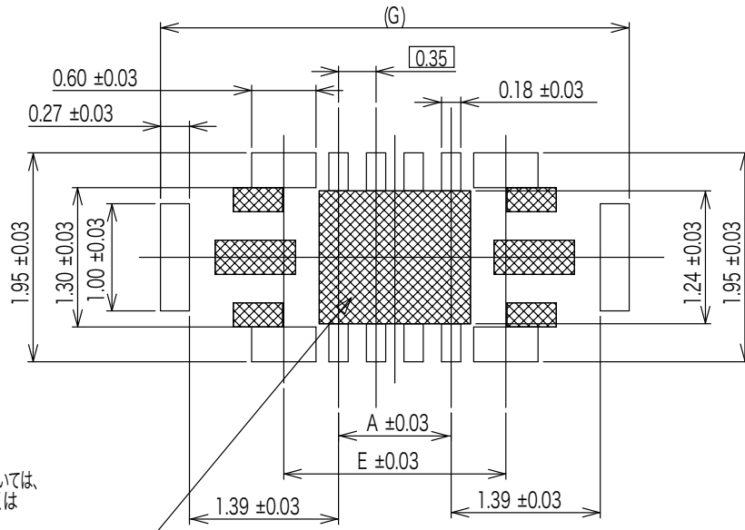
推奨基板寸法
