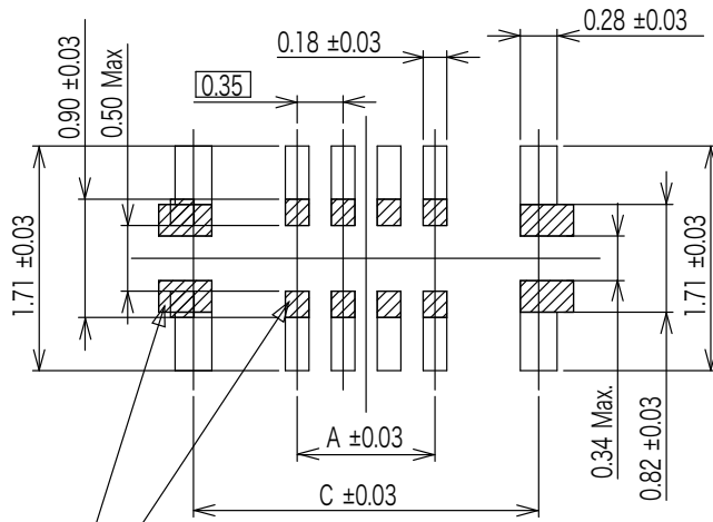
推奨基板寸法
